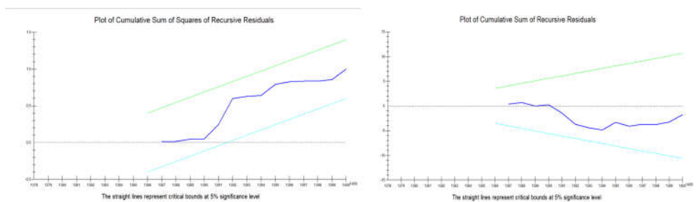
شکل ۱. نمودارهای الف) آزمون CUSUM و ب) آزمون CUSUMSQ مربوط به ثبات ساختاری مدل
